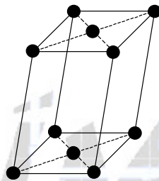
Monoclínico de base centrada (MBC)
