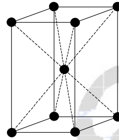
Ortorrômico de corpo centrado (OCC)
