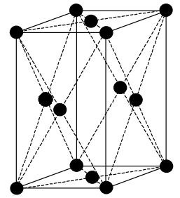
Ortorrômico de face centrada (OFC)
